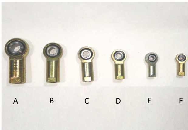
A) # 191-B ARTICULACION OJILLO 1/2 MULTIF. HEMBRA B) # 191-Q ARTICULACION OJILLO 7/16 MULTIF. HEMBRA C) # 191-J ARTICULACION OJILLO 3/8 MULTIF. HEMBRA D) # 191-O ARTICULACION OJILLO 5/16 MULTIF. HEMBRA E) # 191-F ARTICULACION OJILLO 1/4 MULTIF. HEMBRA F) # 191-N
